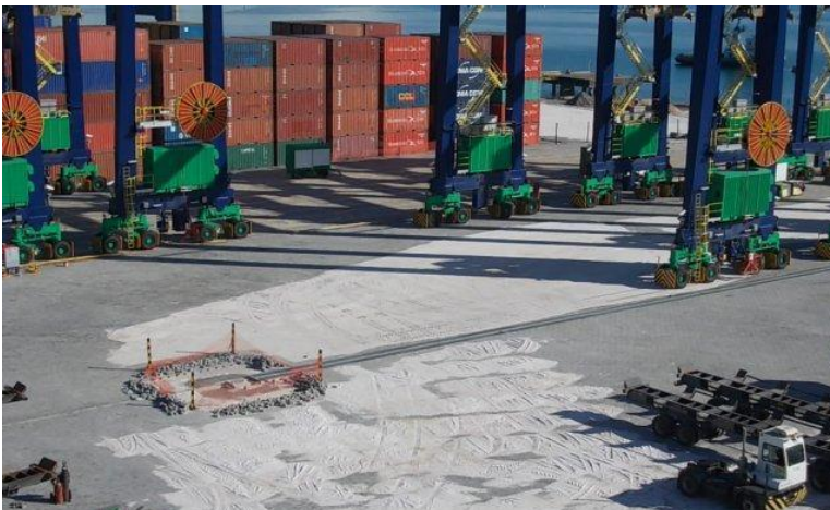
Pavimentação e nivelamento da retro-área (Maio/2012)
